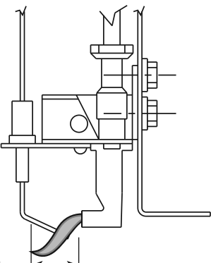
Figure 15.1 - Flamme de veilleuse correcte
